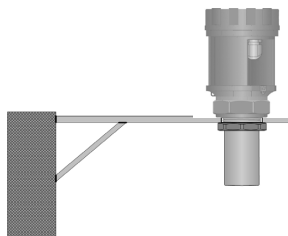
Установка с помощью кронштейна
