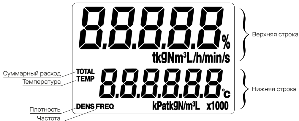
Рис. 4.1 Дисплей расходомера
