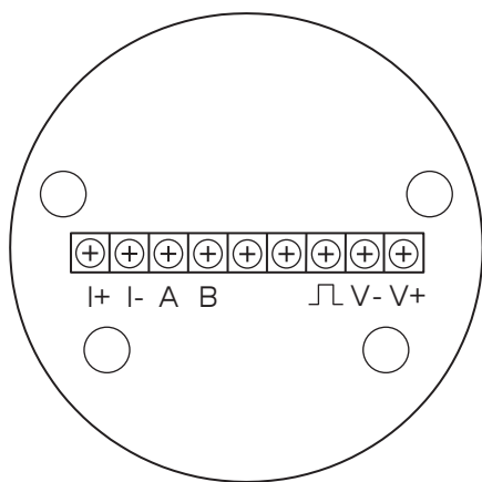
Рис. 3.1. Клеммная колодка
