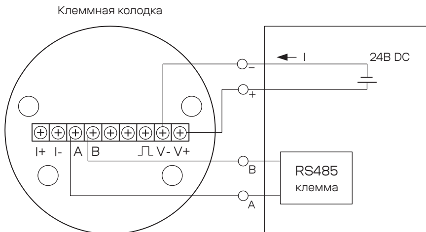
Рис. 3.5. Подключение для RS485
