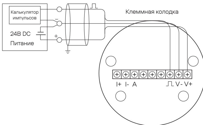
Рис. 3.2. Подключение 3-проводного импульсного выхода
