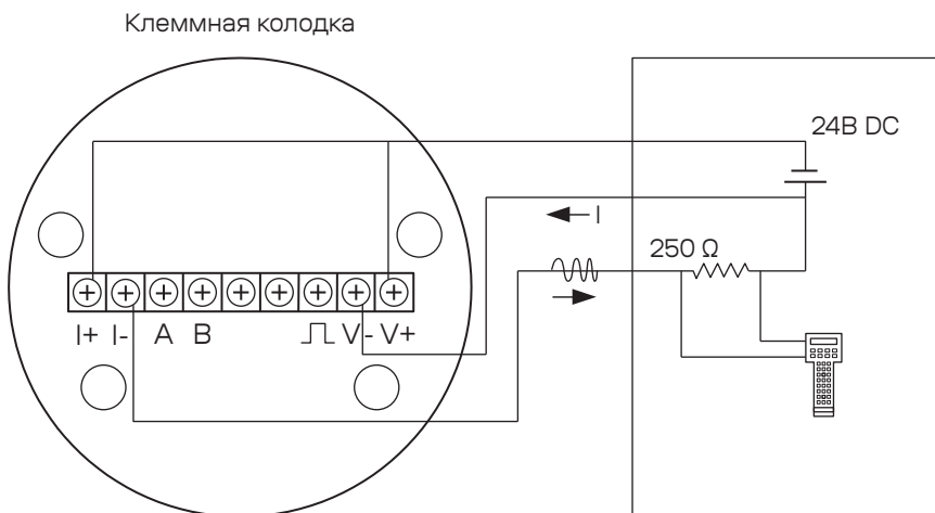
Рис. 3.3. Подключение 3-проводного выхода HART и 4..20 МА
