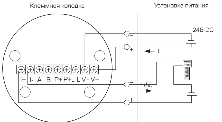
Рис. 3.9. Подключение для RS485 на клеммной колодке AC
